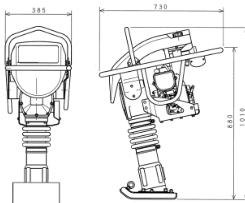
RTX55D/60D外形図、仕様書
